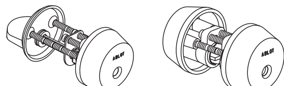
VÄÄNTÖNUPPI + AVAINPESÄ
